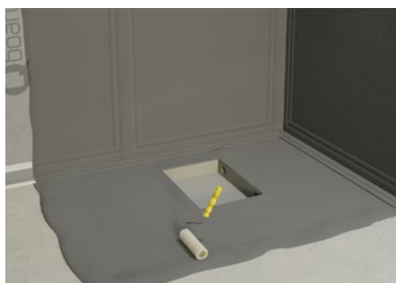
3) Overgangen en oppervlakken afdichten
