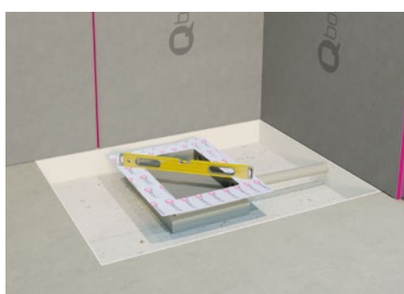
1) De installatiebox uitlijnen en aansluiten
